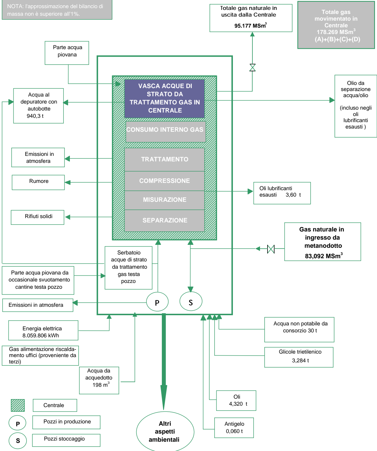
Fig.4 - Bilancio di massa ed energia del Sito di Cellino Attanasio (dati 2014)
