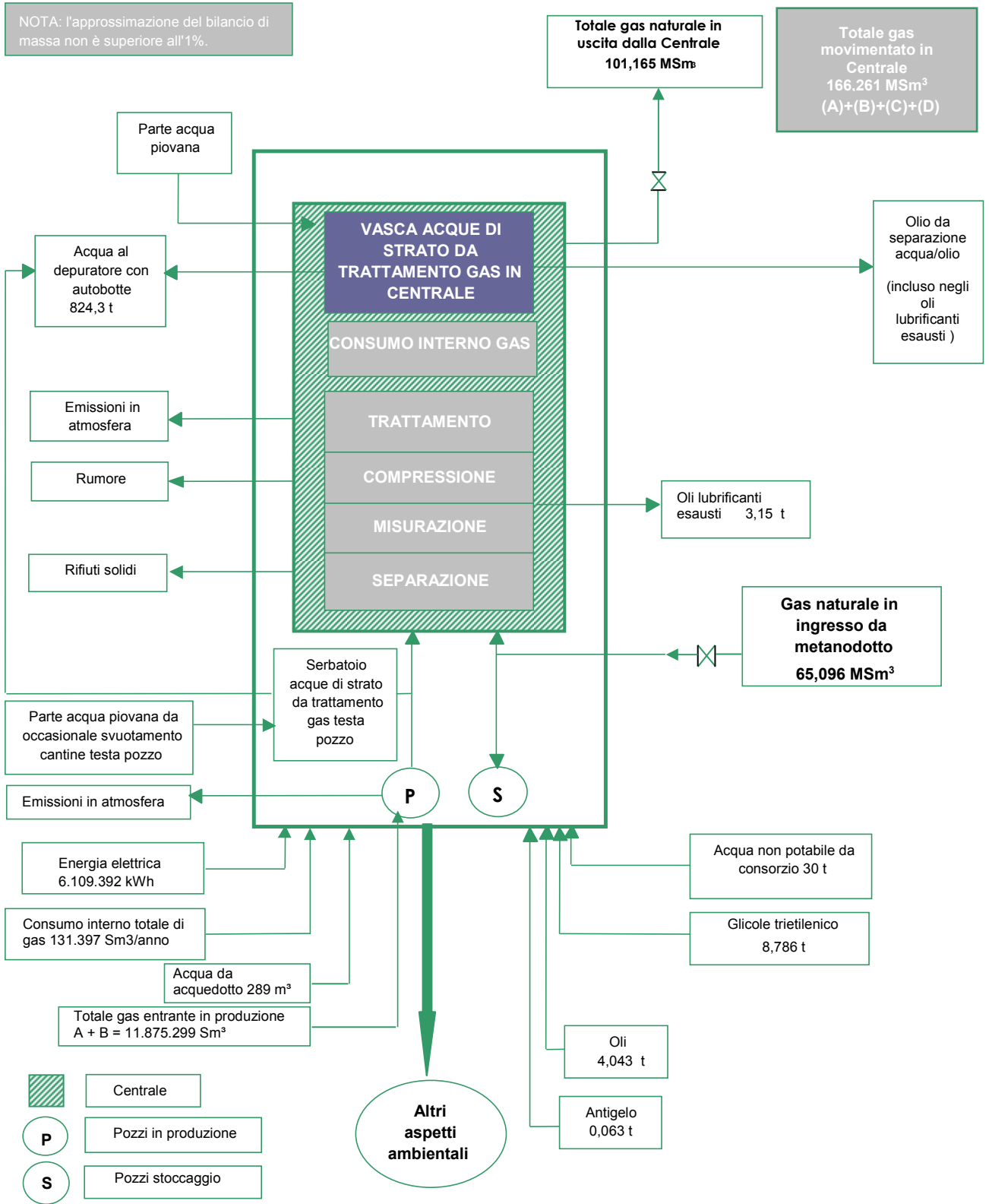
Fig 3 - Bilancio di massa ed energia del Sito di Cellino Attanasio (dati 2016)
