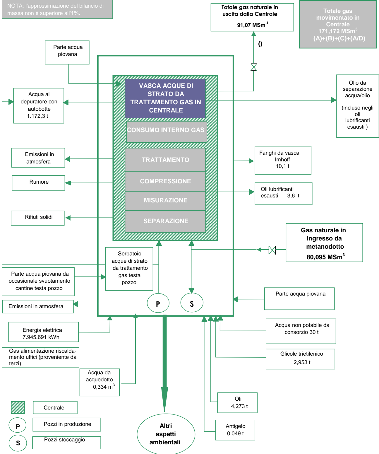
Fig.4 - Bilancio di massa ed energia del Sito di Cellino Attanasio (dati 2012)
